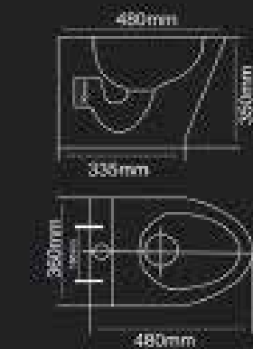
فاسله دو پيچ محل نصب روي فلاش تانگه توکار (180 mm)
